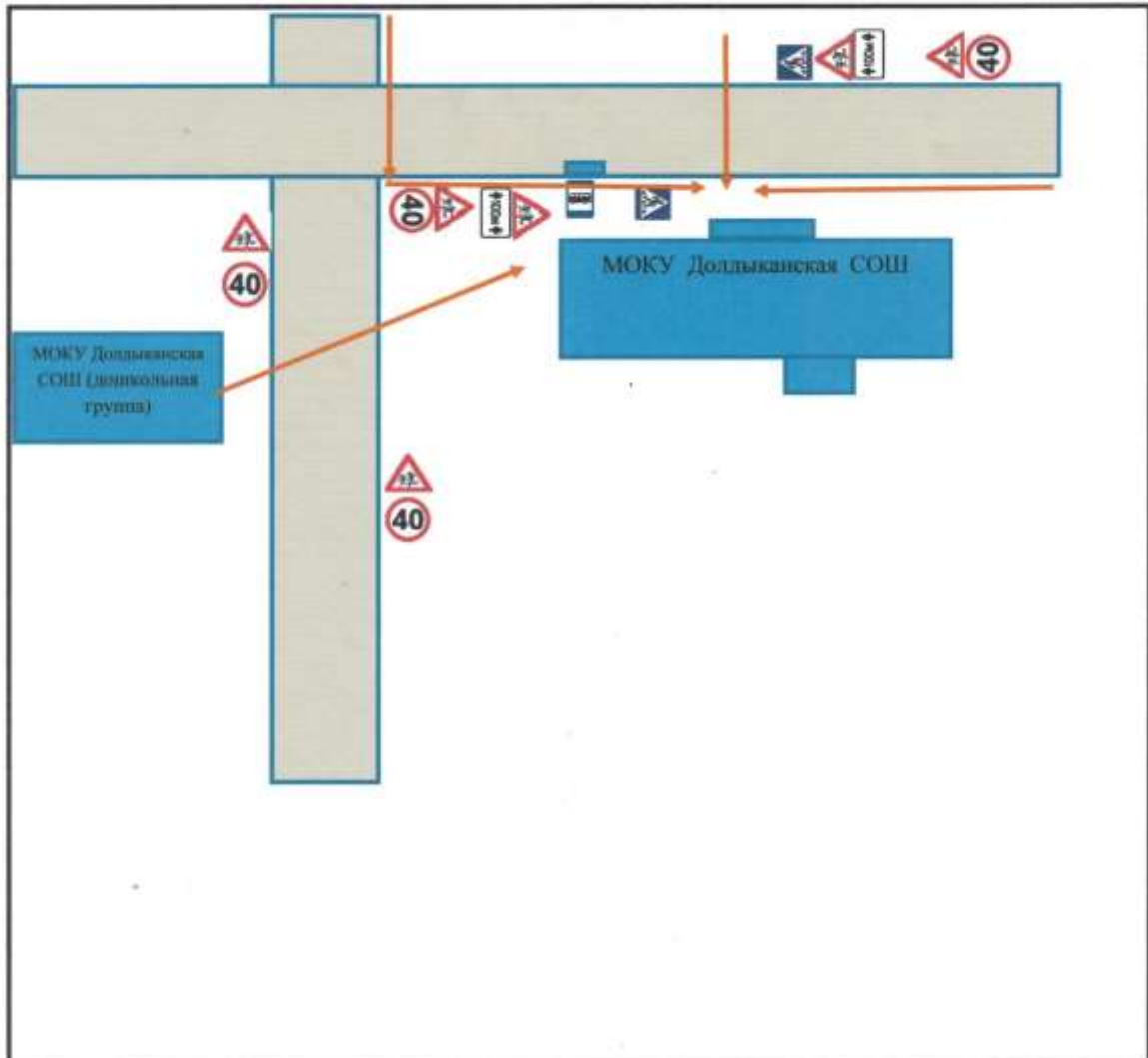
2.Схема организации дорожного движения в непосредственной близости от образовательного учреждения с размещением соответствующих технических средств организации дорожного движения, маршрутов движения детей и расположения парковочных мест.
